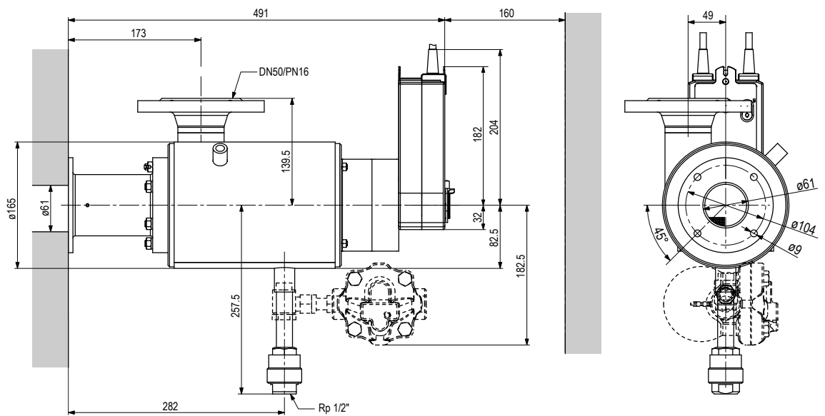
Silownik CA150A-MP / CA150A-S Condair Esco 20 stal nierdzewna
