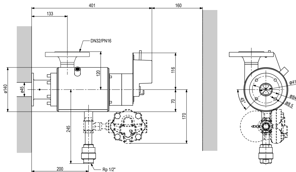
Siłownik CA75 Condair Esco 10 stal nierdzewna
