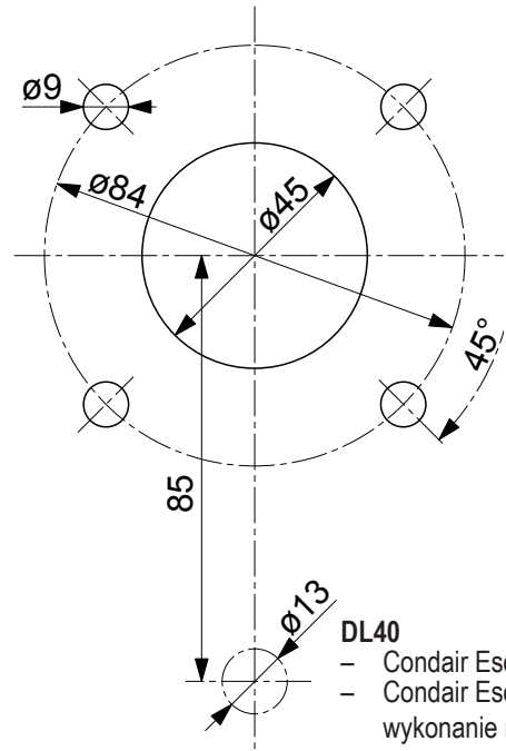
DR73 - Condair Esco 10 wykonanie nierdzewne
