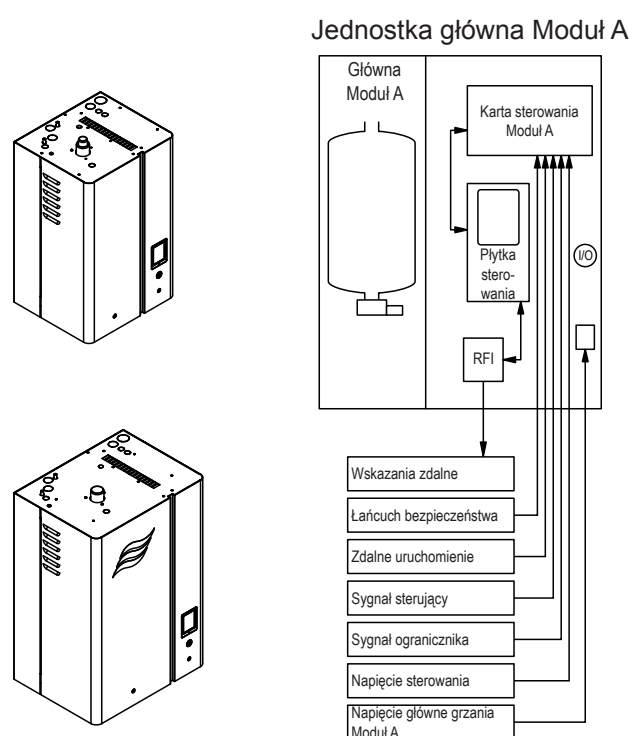
Fig. 1: Pojedyncze jednostki małe ("S") i średnie ("M")
