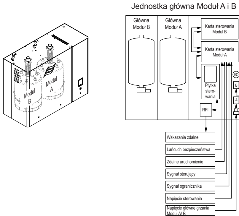
Fig. 2: Pojedyncze jednostki duże ("L")
