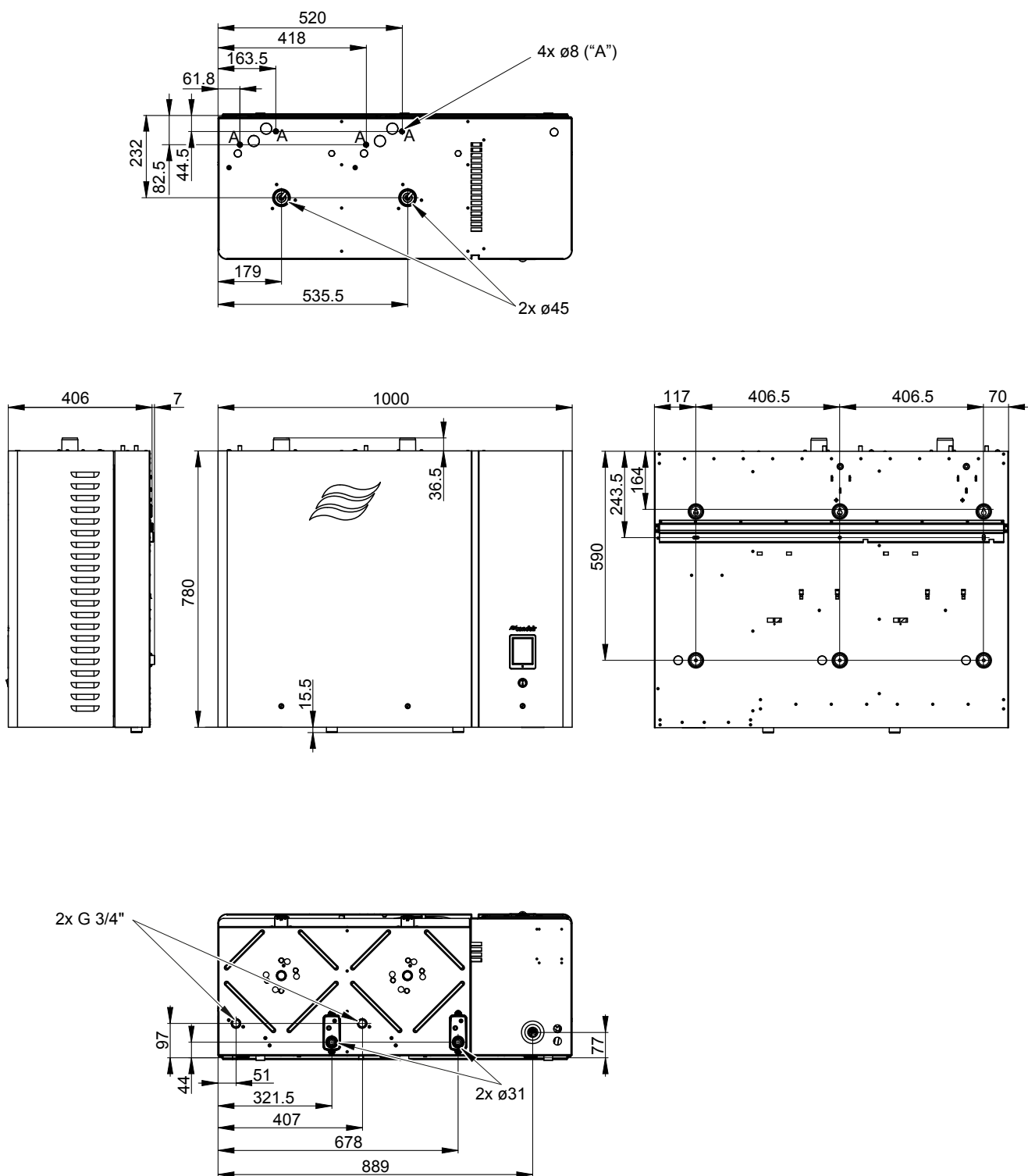
Fig. 31: Wymiary jednostek Condair EL 50-90, wielkość "S" (wymiary w mm)
