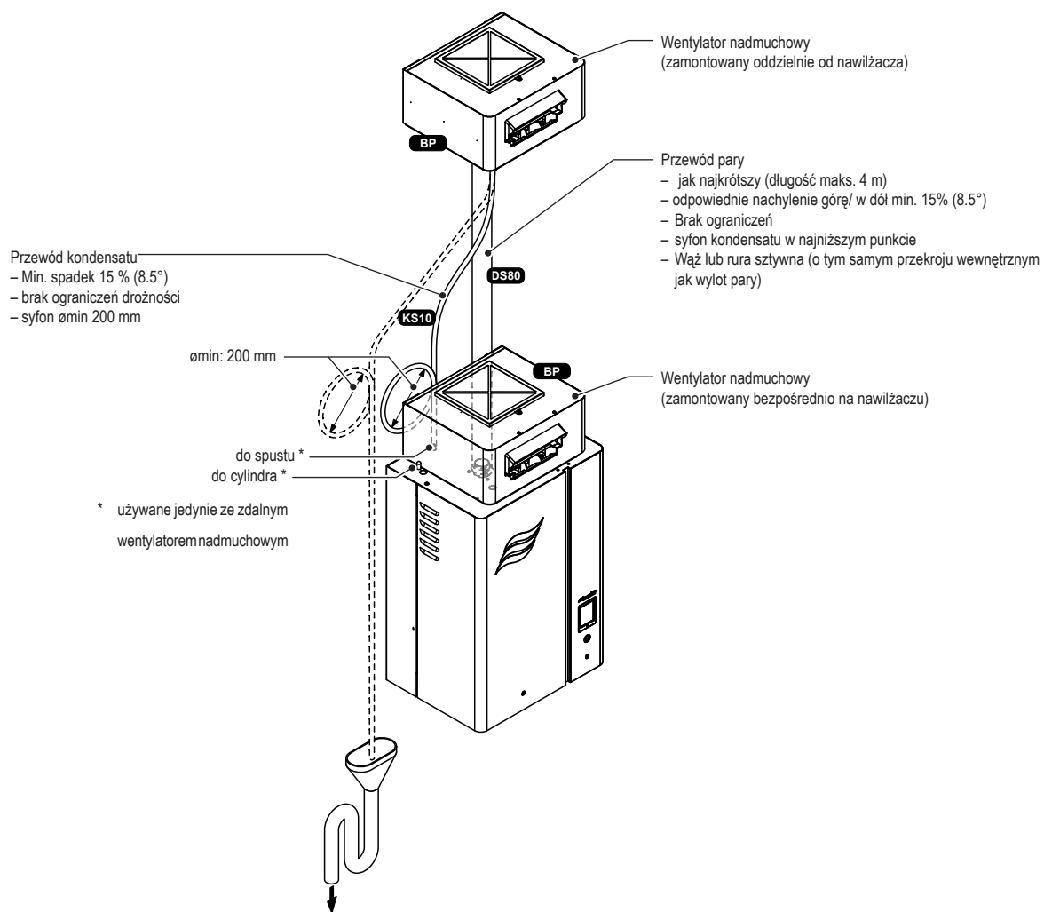
Fig. 13: Instalacja do nawilżania pomieszczeń
