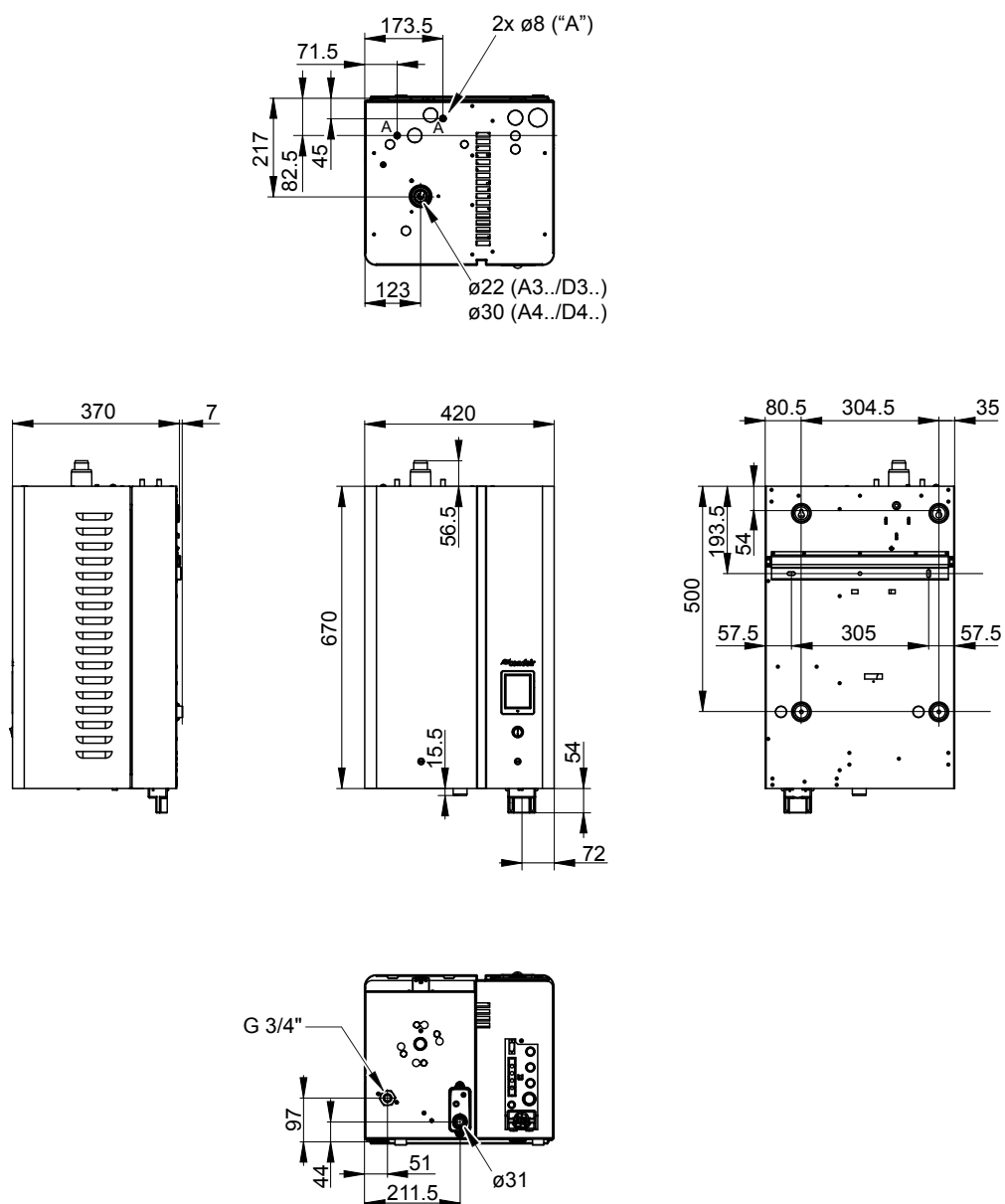
Fig. 29: Wymiary jednostek Condair EL 5 - 15, wielkość "S" (wymiar w mm)
