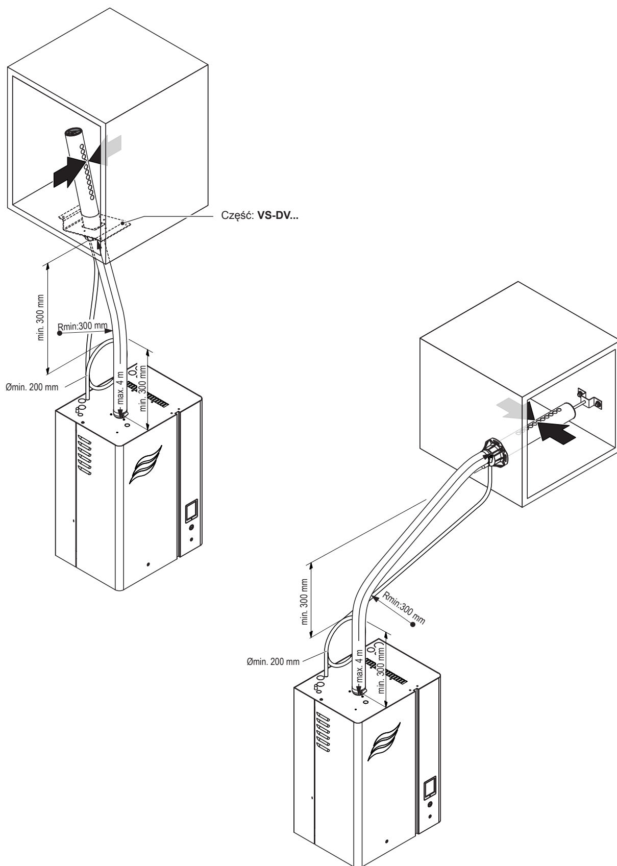
Fig. 15: Lanca parowa zamontowana więcej niż 500 mm nad krawędzią nawilzacza
