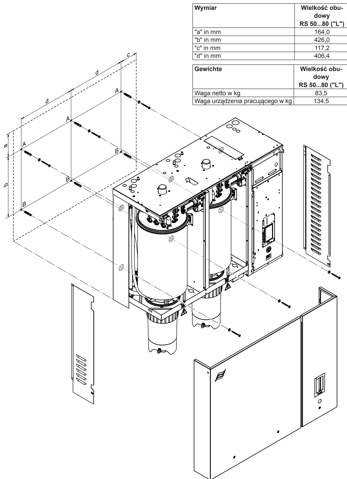
Rys. 12: Przegląd standardowego montażu dużych ("L") jednostek
