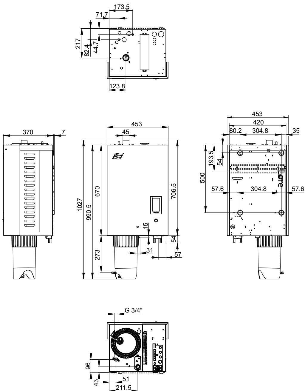
Rys. 34: Rysunek wymiarowy, jednostka mała ("S") (wymiar w mm)
