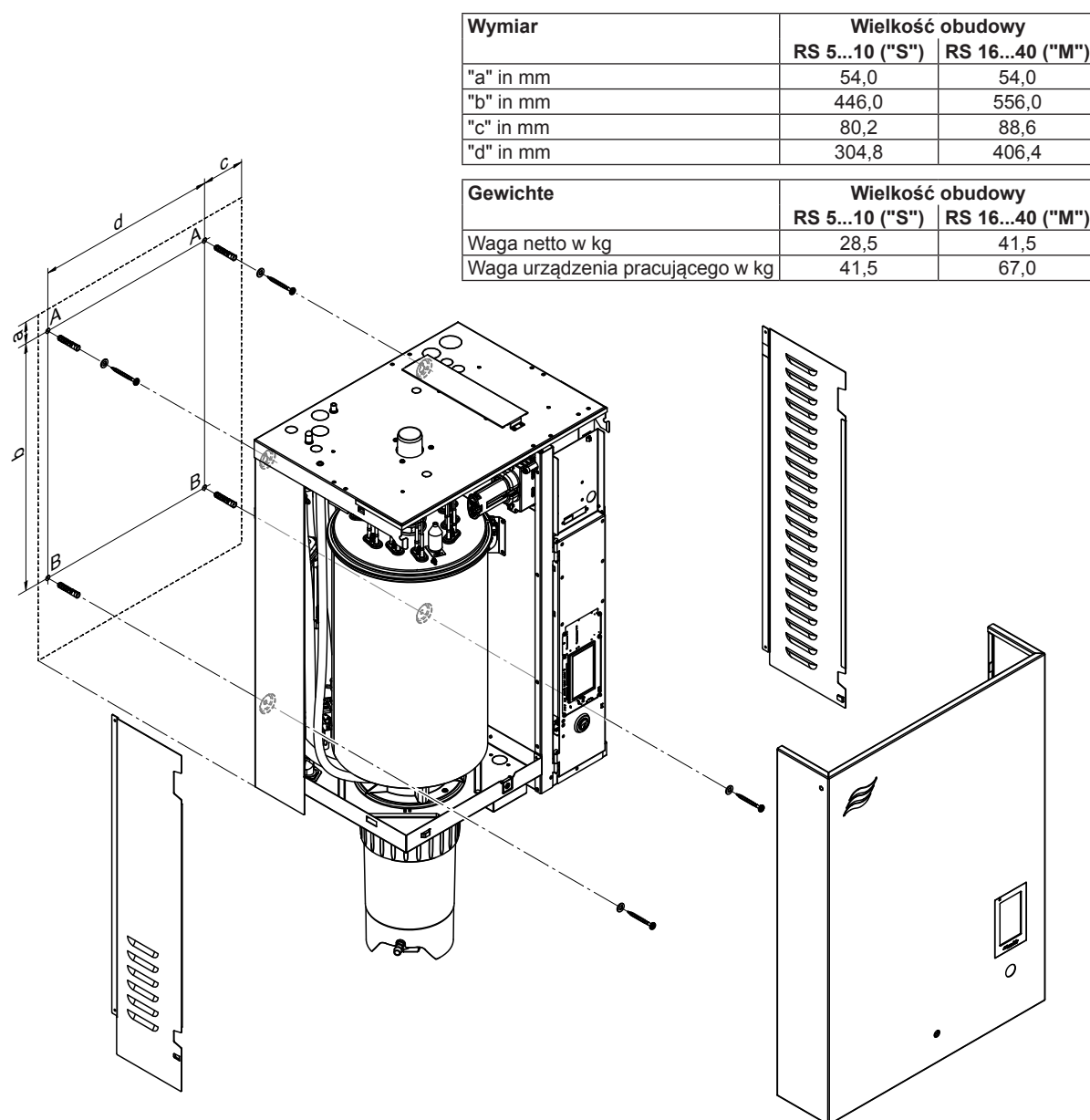
Rys. 11: Przegląd standardowego montażu małych ("S") i średnich ("M") jednostek
