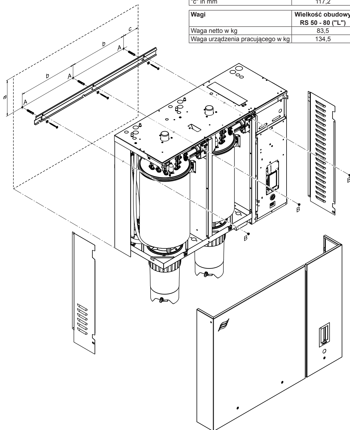
Rys. 14: Przegląd montażu dużych ("L") jednostek z szyną montażową
