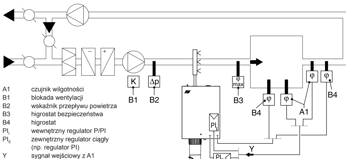
Rys. 25: System 1 – regulacja wilgotności w pomieszczeniu
