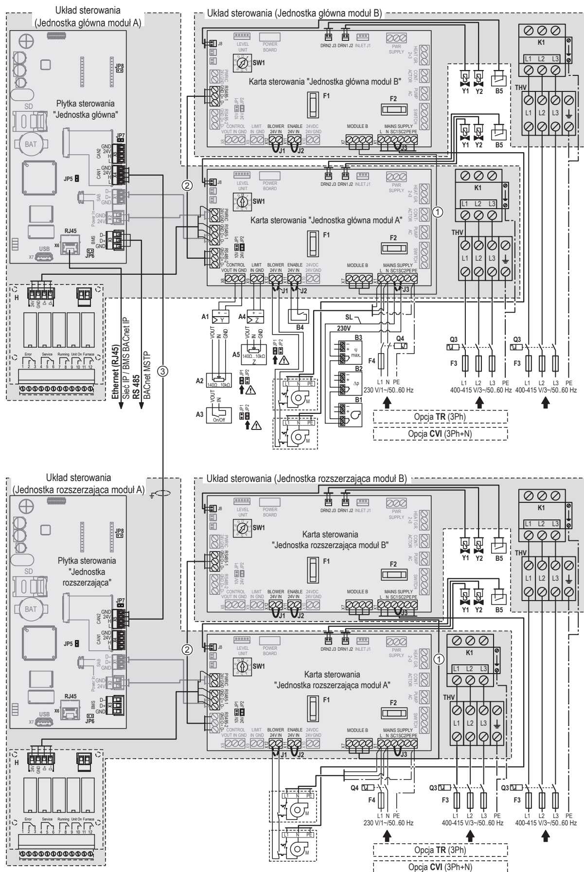
Rys. 31: Schemat połączeń RS 100...160 - System połączonych urządzeń 3 x "M" lub 4 x "M"
