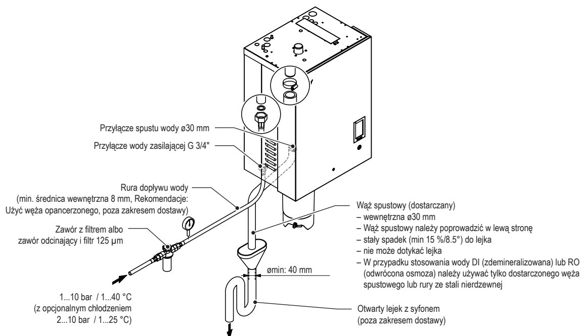
Rys. 22: Widok ogólny instalacji wodnej dla jednostek małych ("S") i średnich ("M")
