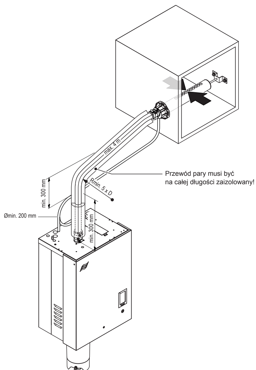
Rys. 20: Sztywne przewody rurowe pary, zaizolowane
