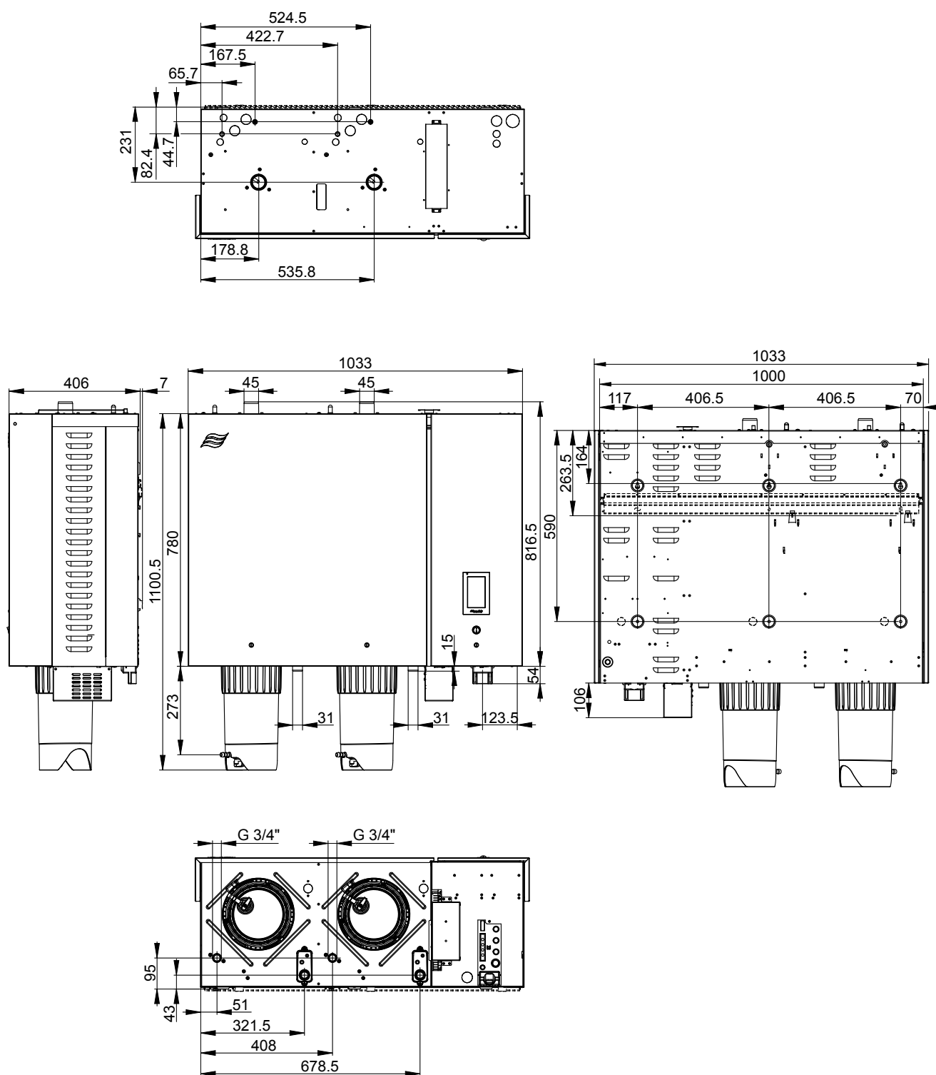
Rys. 36: Rysunek wymiarowy, jednostka duża ("L") (wymiary w mm)
