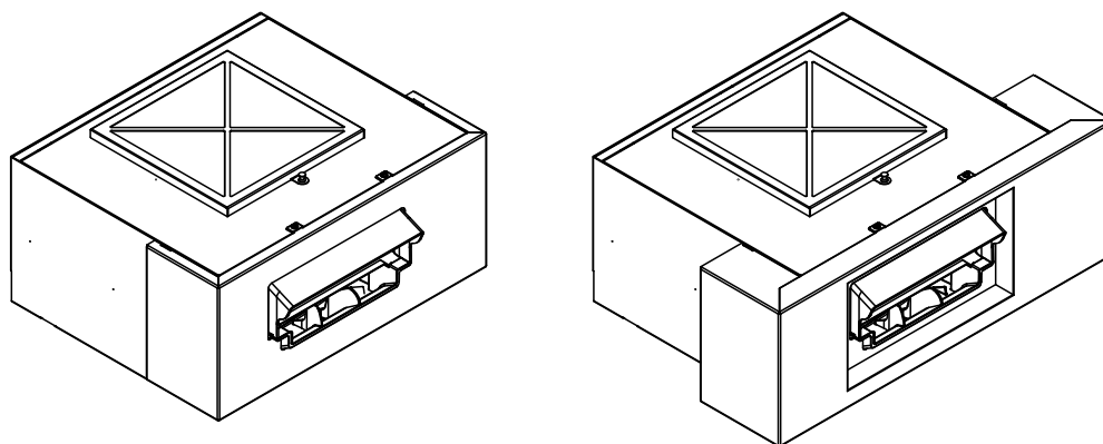
Rys. 7: Wentylatory nadmuchowe z małą osłoną (po lewej) i dużą osłoną (po prawej)
