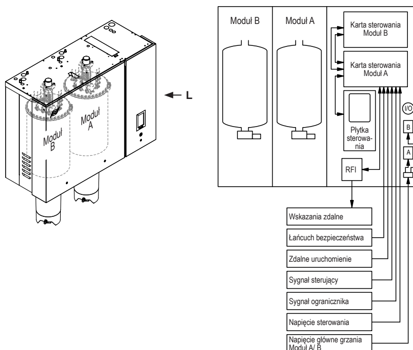
Rys. 2: Pojedyncze jednostki duże ("L")
