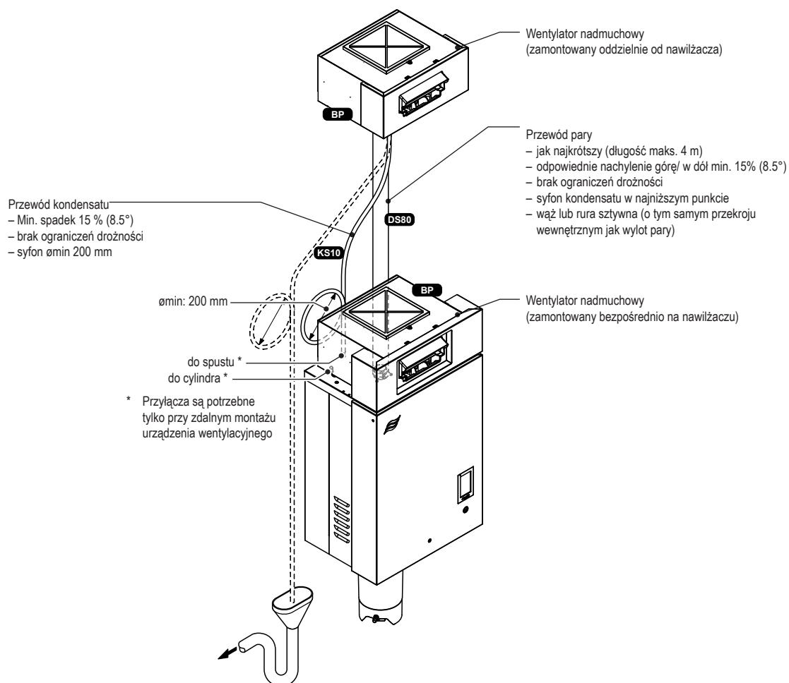
Rys. 16: Instalacja do nawilżania pomieszczeń
