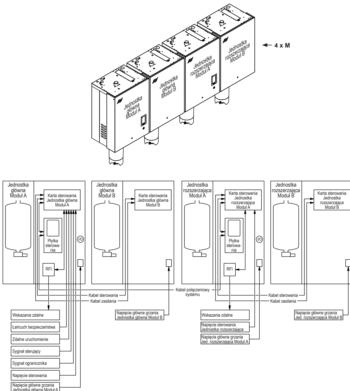
Rys. 5: Systemy połączonych urządzeń (4 x "M")
