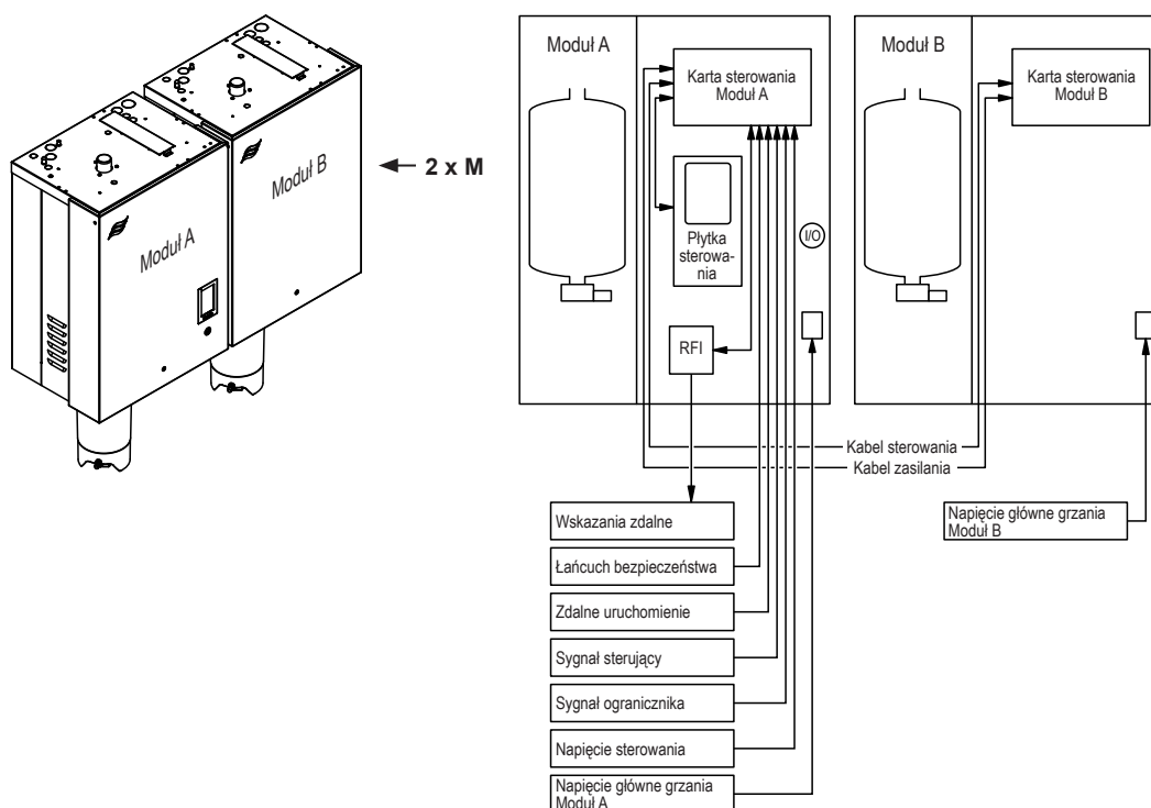
Rys. 3: Jednostki podwójne (2 x "M")
