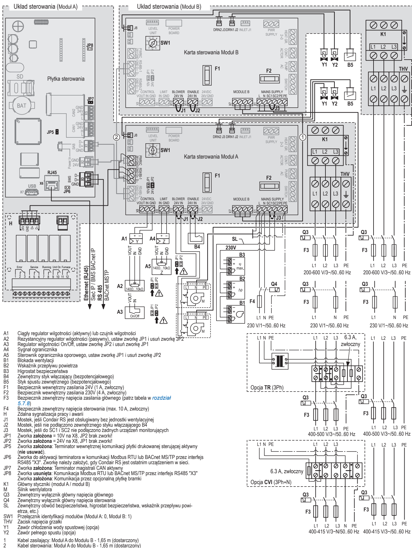
Rys. 30: Schemat połączeń Condair RS 40...80 - jednostki podwójne (2 x pojedyncze obudowy "M")
