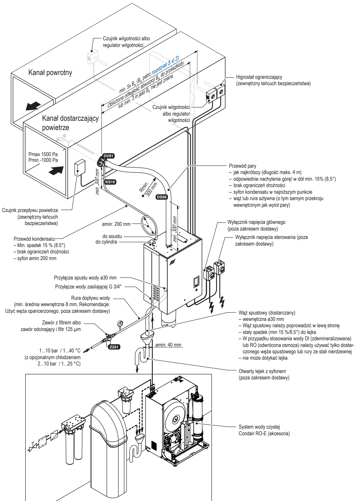
Rys. 8: Typowa instalacja do nawilżania kanałowego
