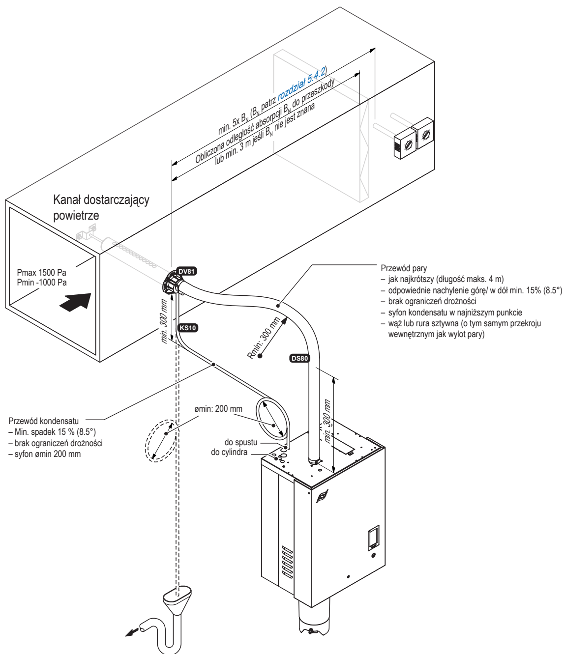
Rys. 15: Instalacja do nawilżania kanałowego
