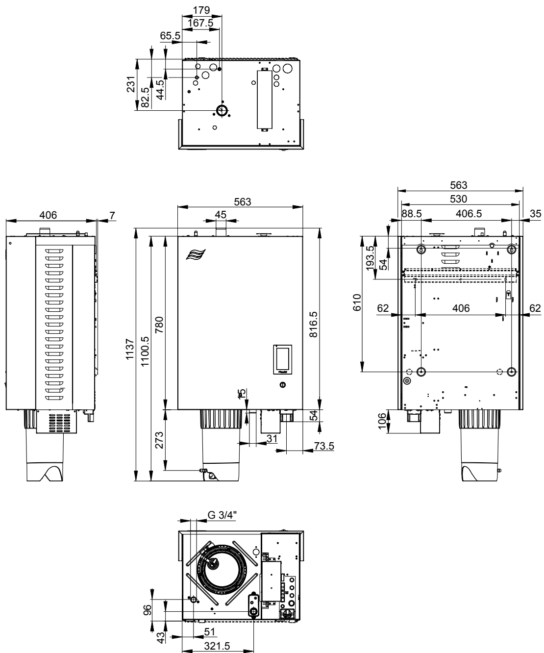
Rys. 35: Rysunek wymiarowy, jednostka średnia ("M") (wymiary w mm)
