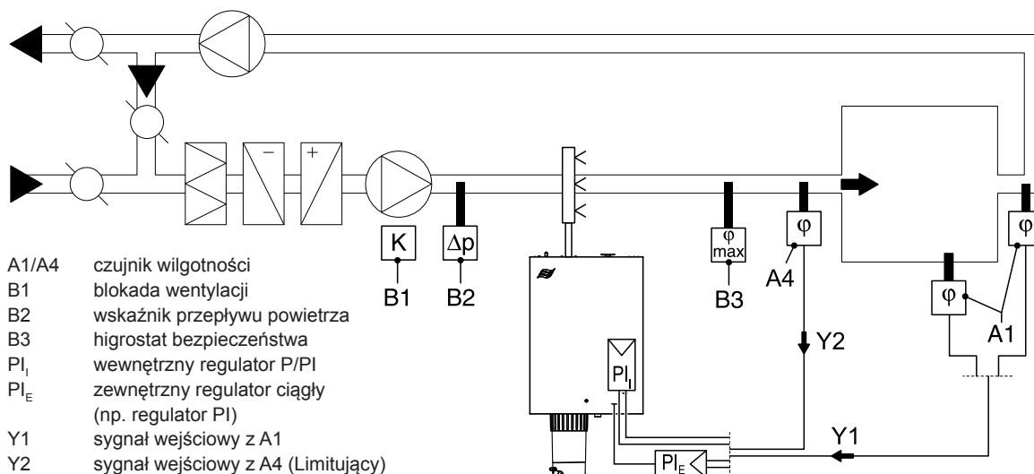
Rys. 26: System 2 – regulacja wilgotności w pomieszczeniu z ciągłym ograniczaniem wilgotności powietrza nawiewanego
