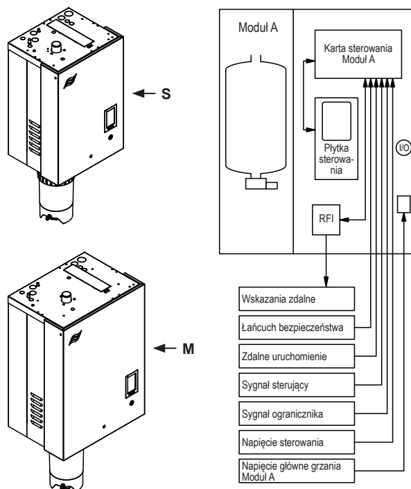
Rys. 1: Pojedyncze jednostki małe ("S") i średnie ("M")
