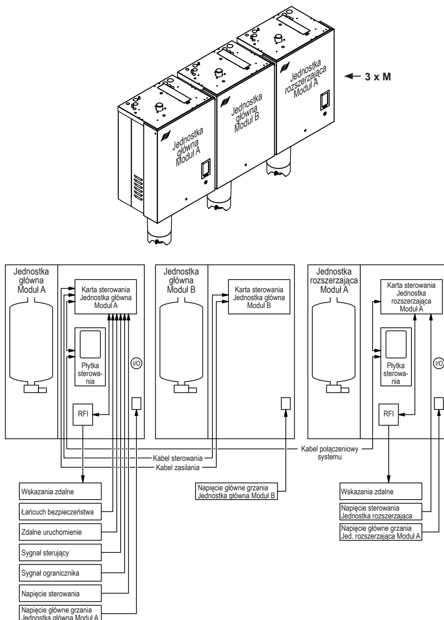
Rys. 4: Systemy połączonych urządzeń (3 x "M")
