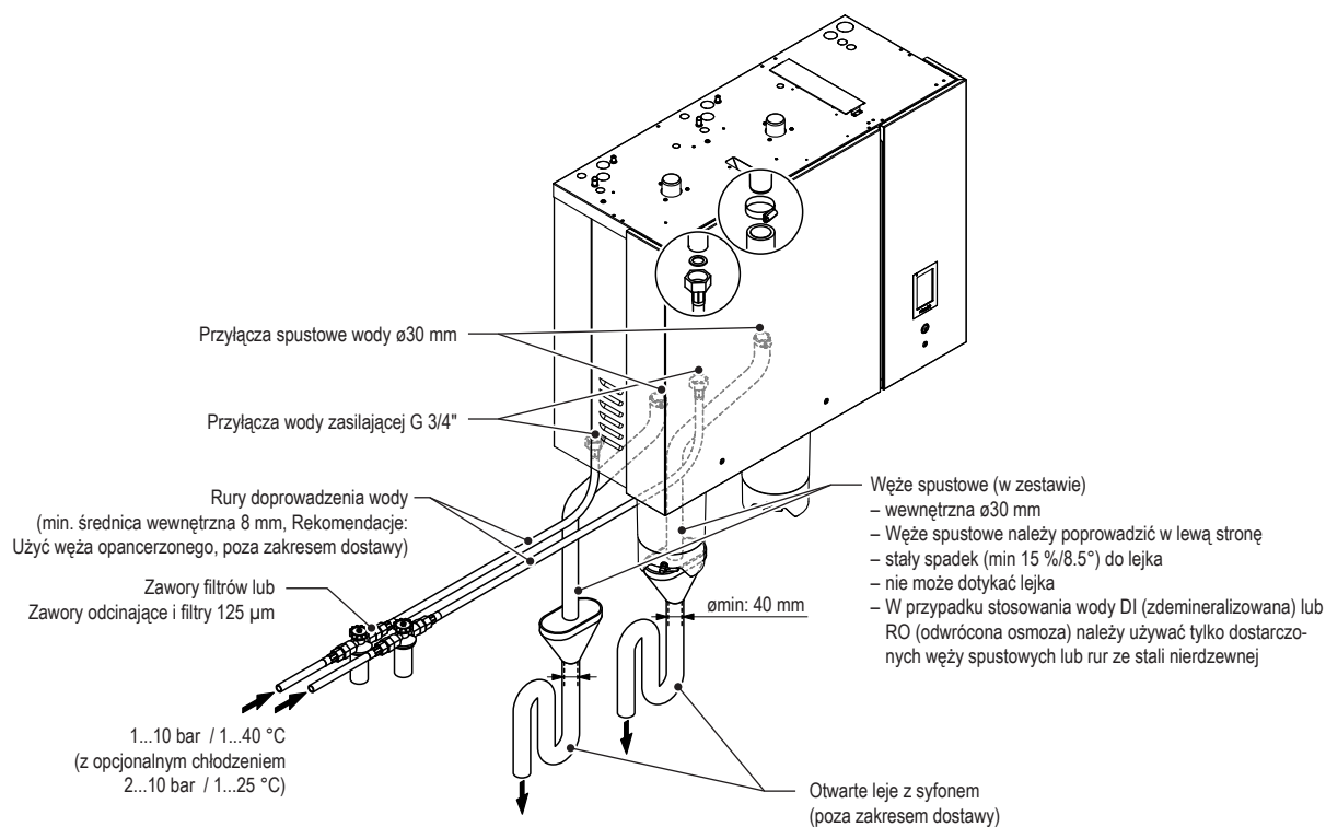
Rys. 23: Widok ogólny instalacji wodnej dla jednostek dużych ("L")
