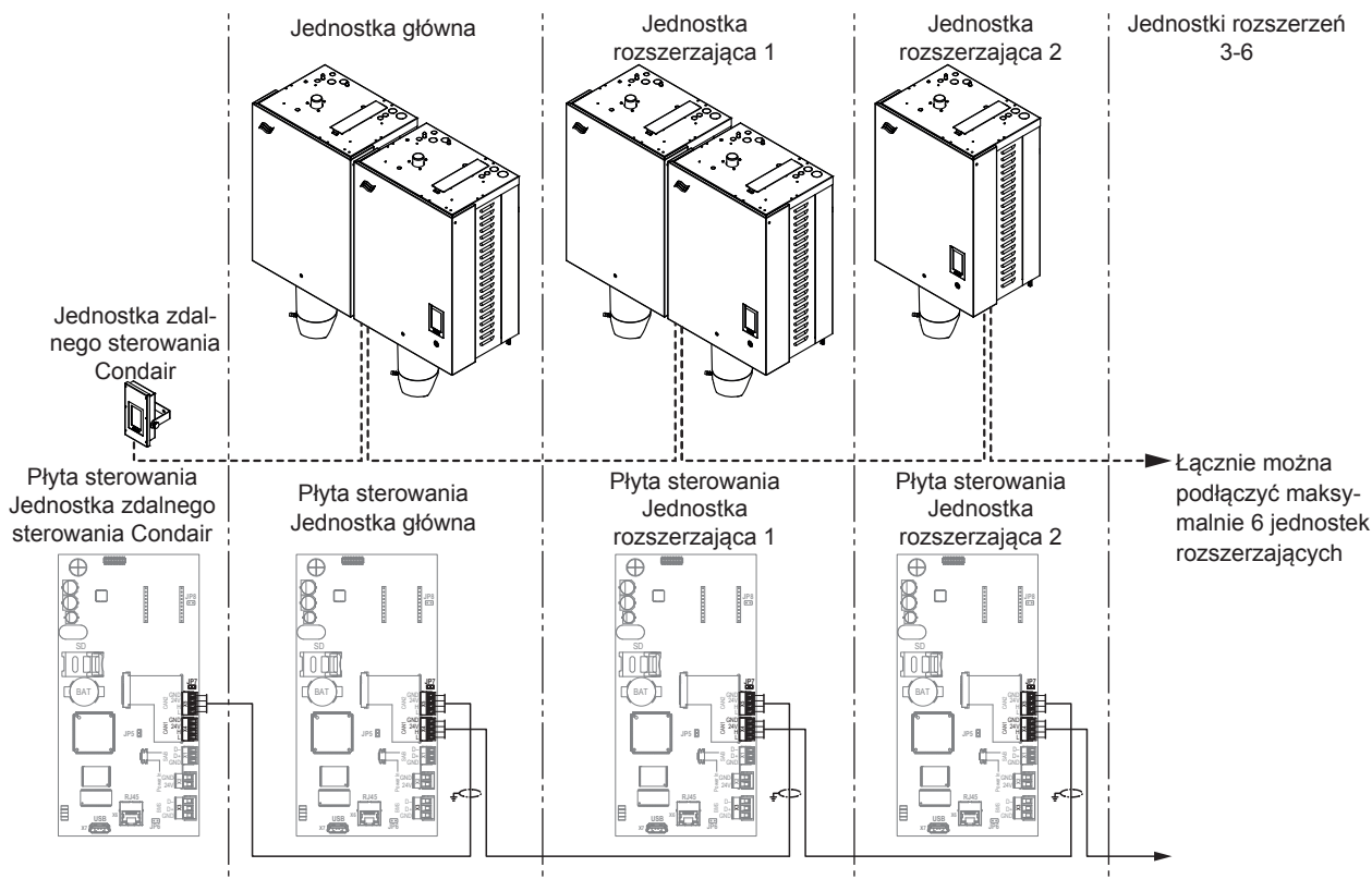
Rys. 32: Łączenie wielu urządzeń (system połączonych urządzeń)
