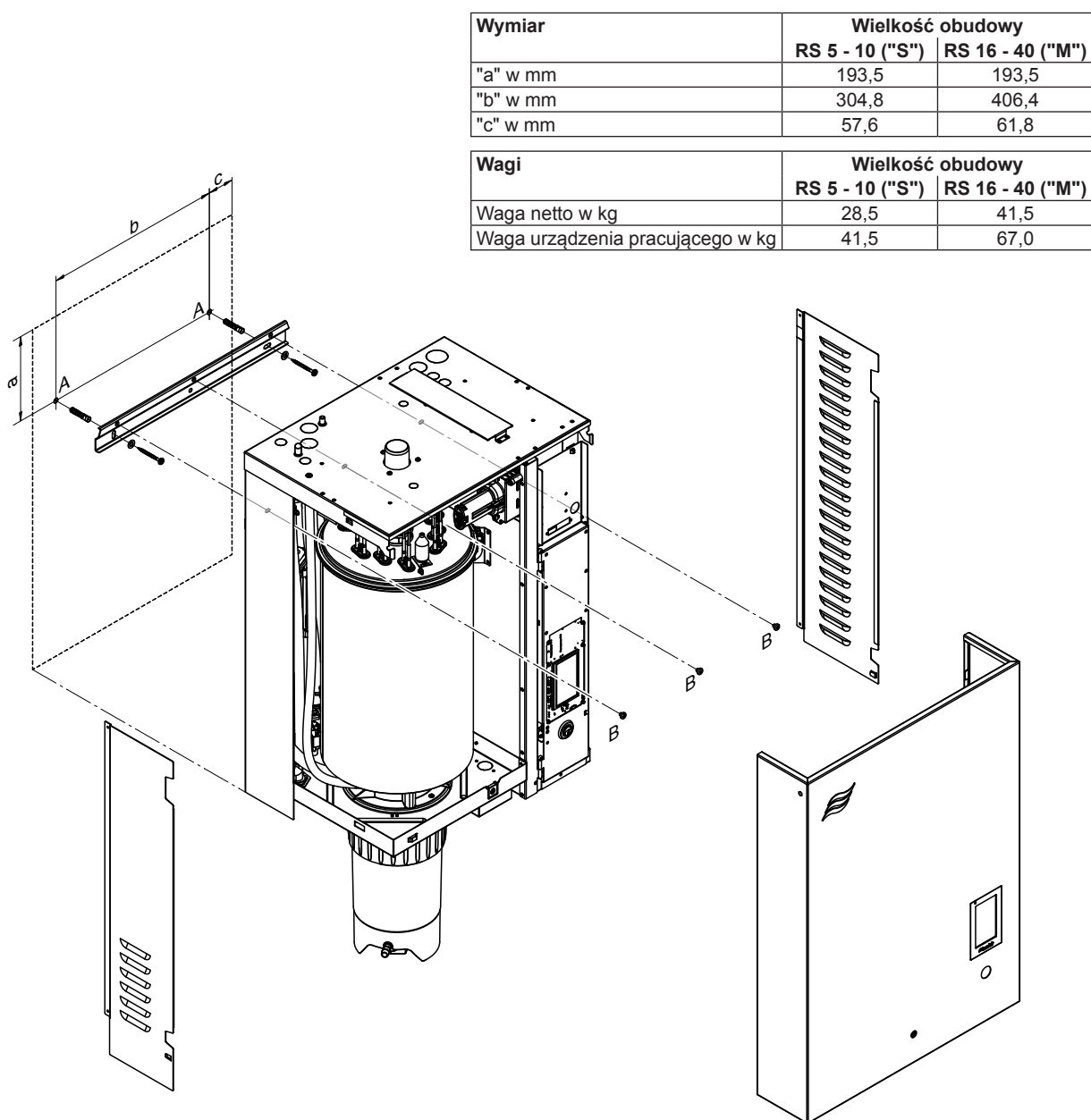
Rys. 13: Przegląd montażu jednostek małych ("S") i średnich ("M") jednostek z szyną montażową
