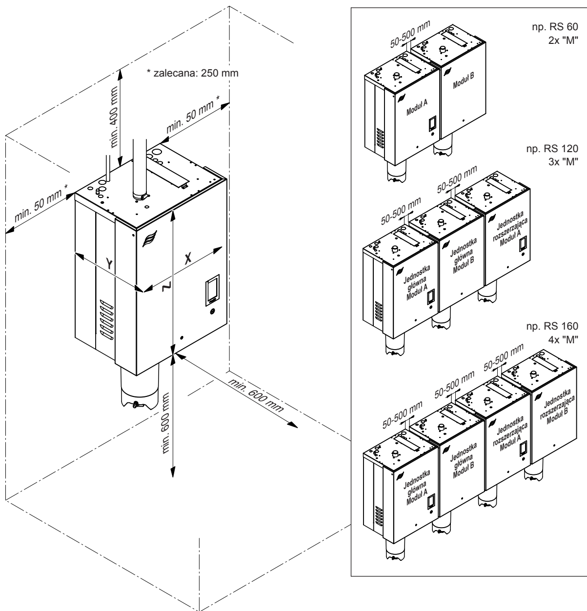
Rys. 10: Odległości, które trzeba zachować
