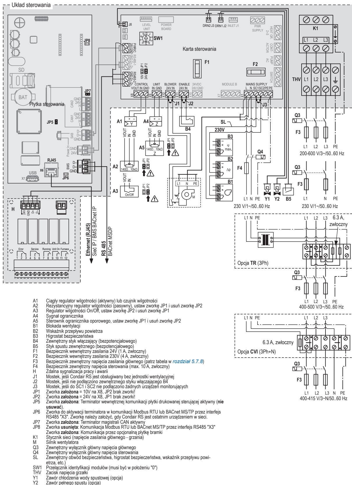
Rys. 28: Schemat połączeń Condair RS 5...40 - jednostki pojedyncze "S" i "M"
