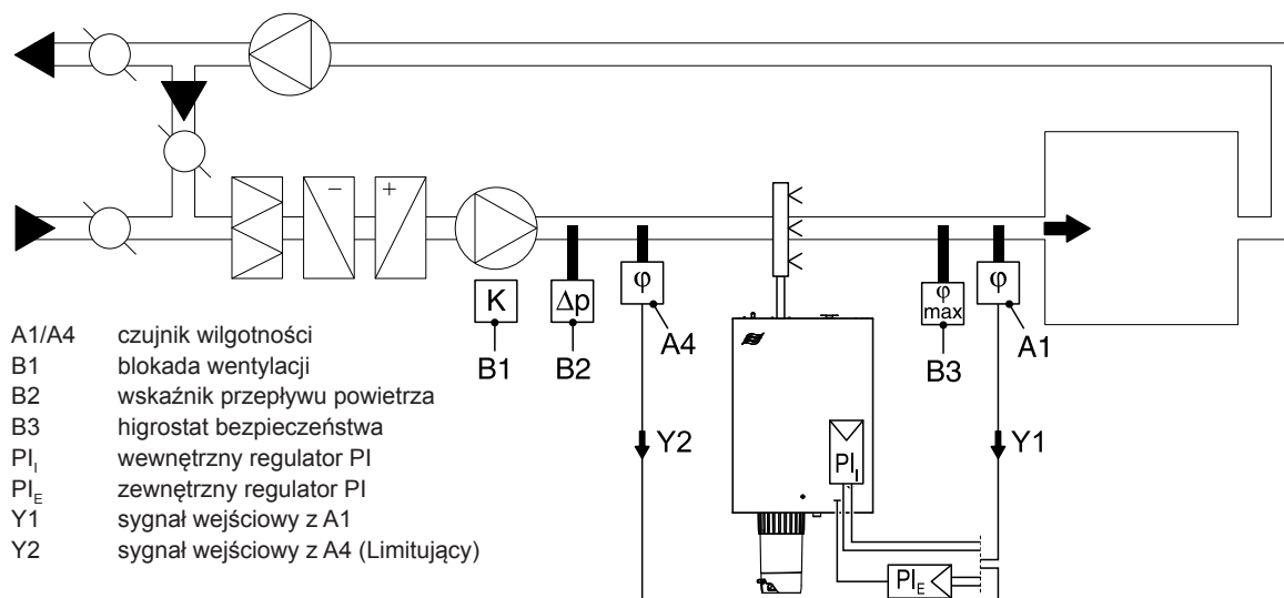
Rys. 27: System 3 – regulacja wilgotności w pomieszczeniu z ciągłym ograniczaniem wilgotności powietrza nawiewanego
