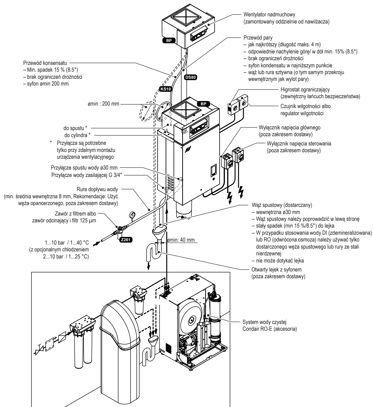
Rys. 9: Typowa instalacja do nawilżania pomieszczeń
