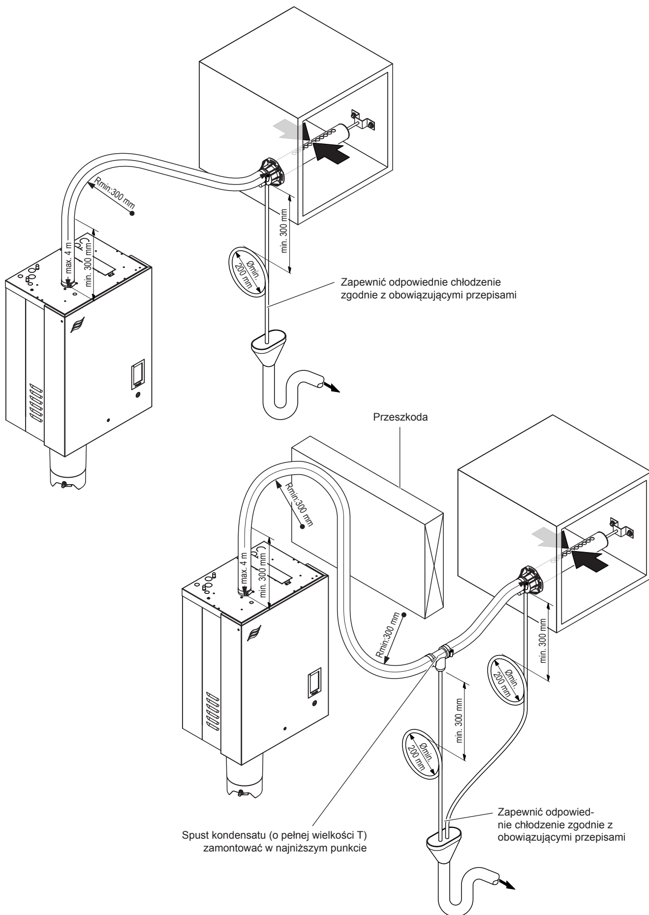
Rys. 19: Lanca parowa zamontowana mniej niż 500 mm nad krawędzią nawilżacza
