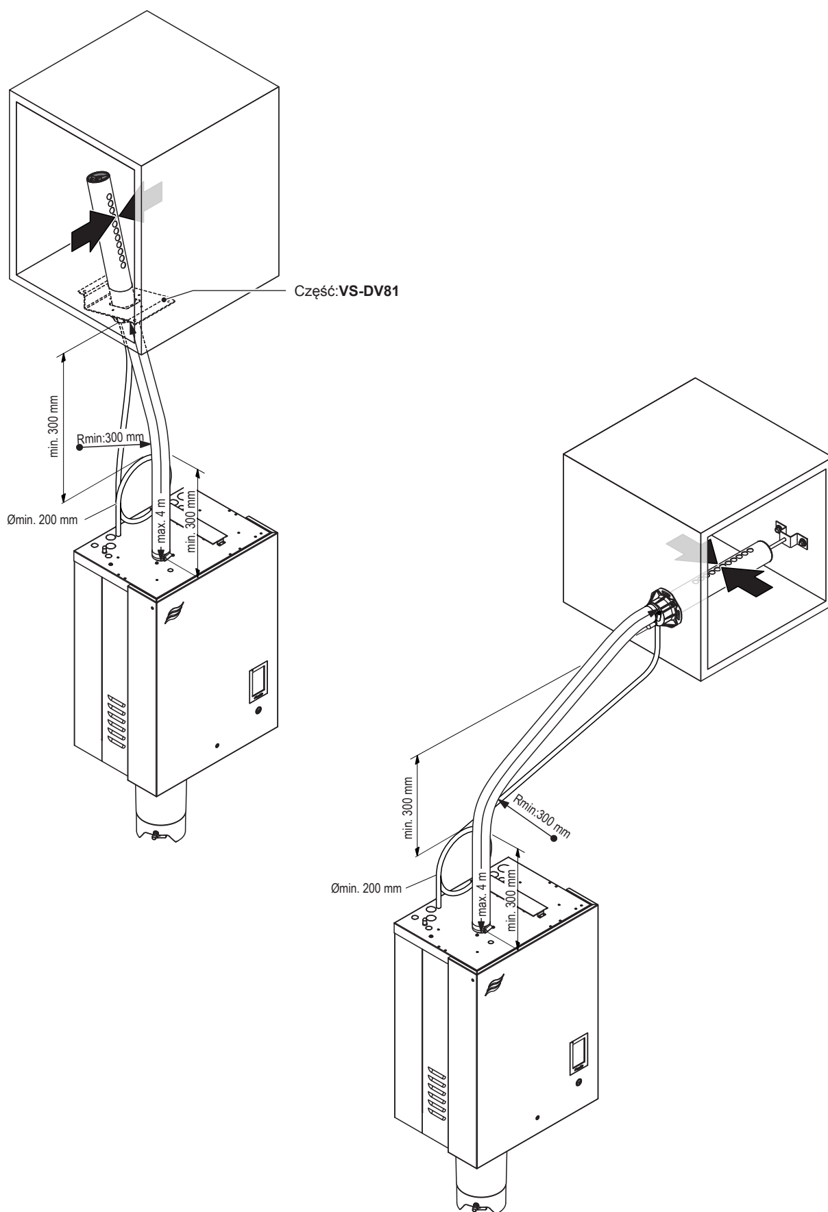
Rys. 18: Lanca parowa zamontowana więcej niż 500 mm nad krawędzią nawilzacza
