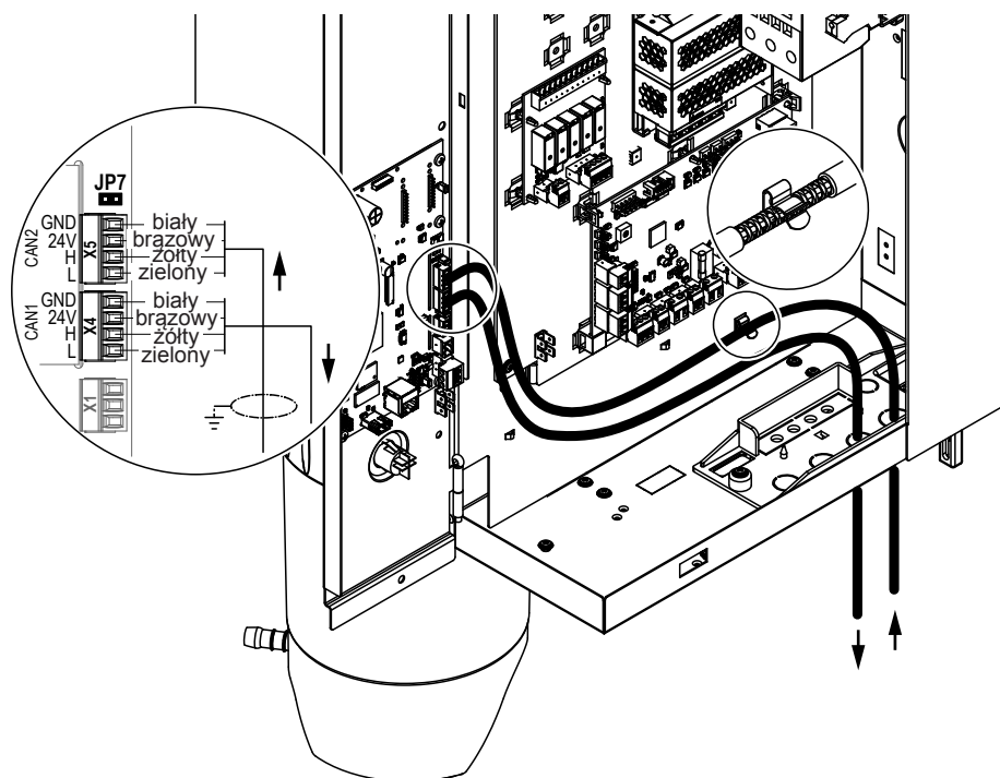
Rys. 33: Przyłącze kabla magistrali CAN / ekranowanie
