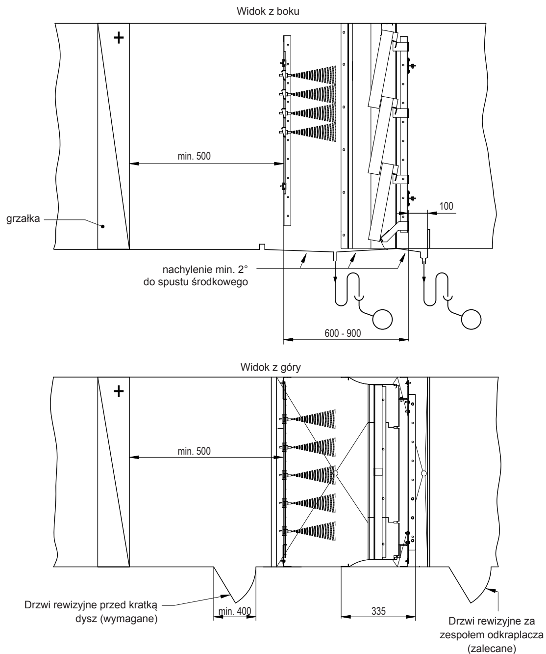
Rys. 3: Umieszczenie nawilżacza z drzwiami rewizyjnymi przed i za nawilżaczem: wymiary w mm
