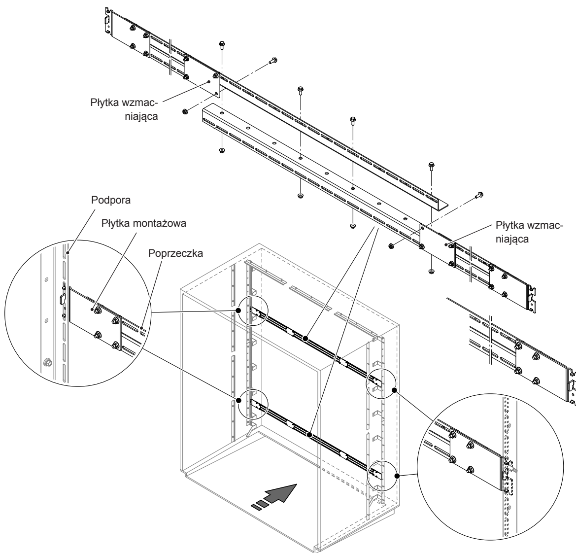
Rys. 10: Montaż poprzeczek
