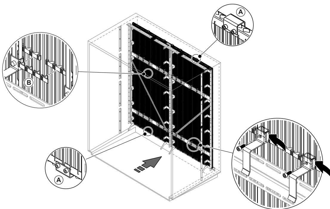
Rys. 17: Montaż elementów odkraplacza
