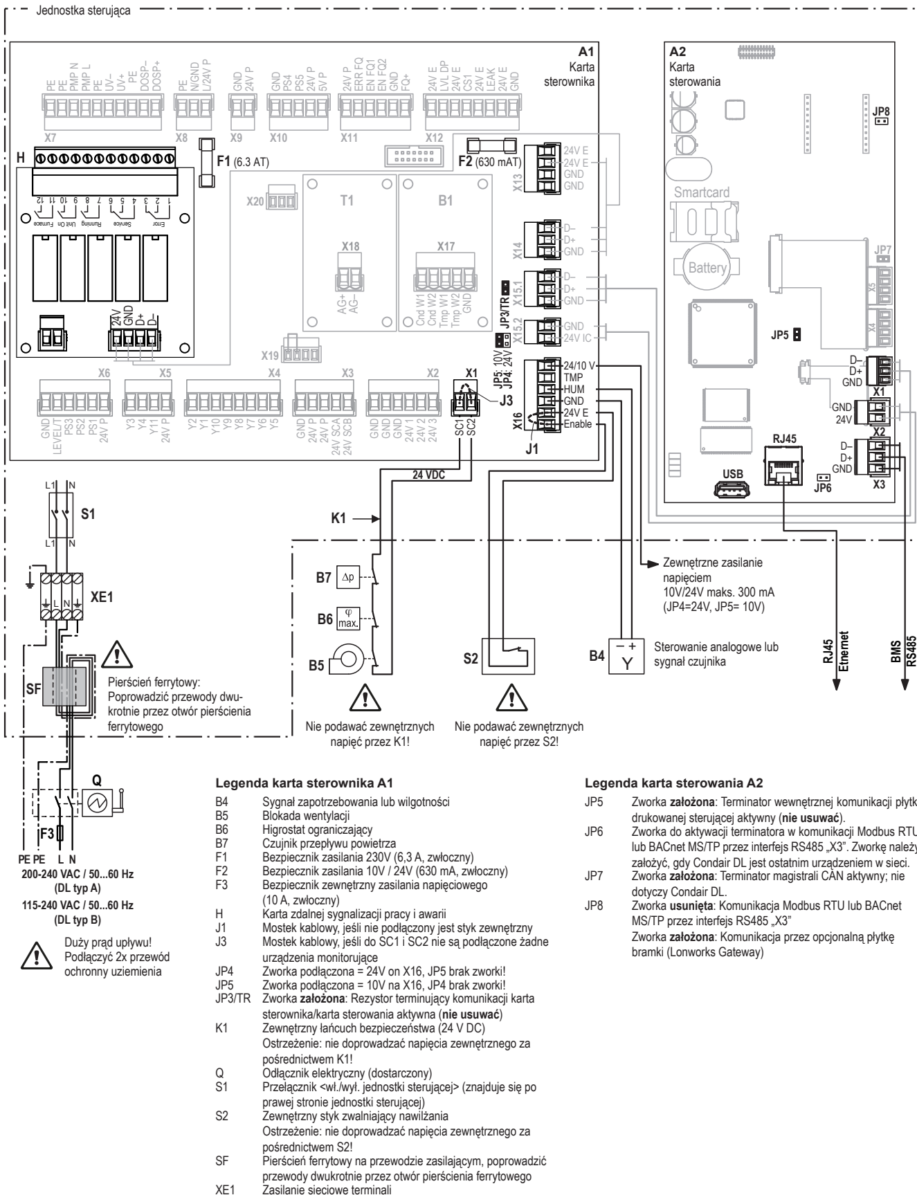
Rys. 40: Schemat zewnętrznych połączeń elektrycznych
