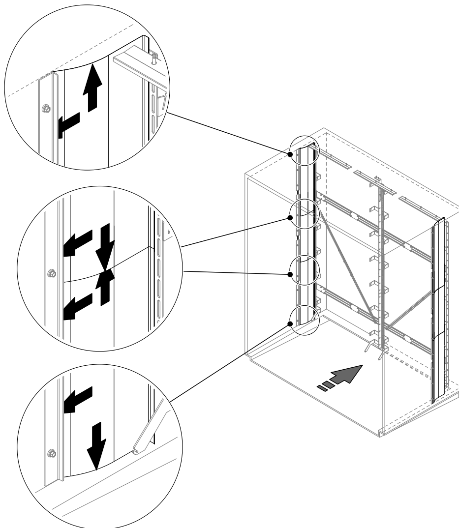
Rys. 18: Montaż bocznych płyt uszczelniających
