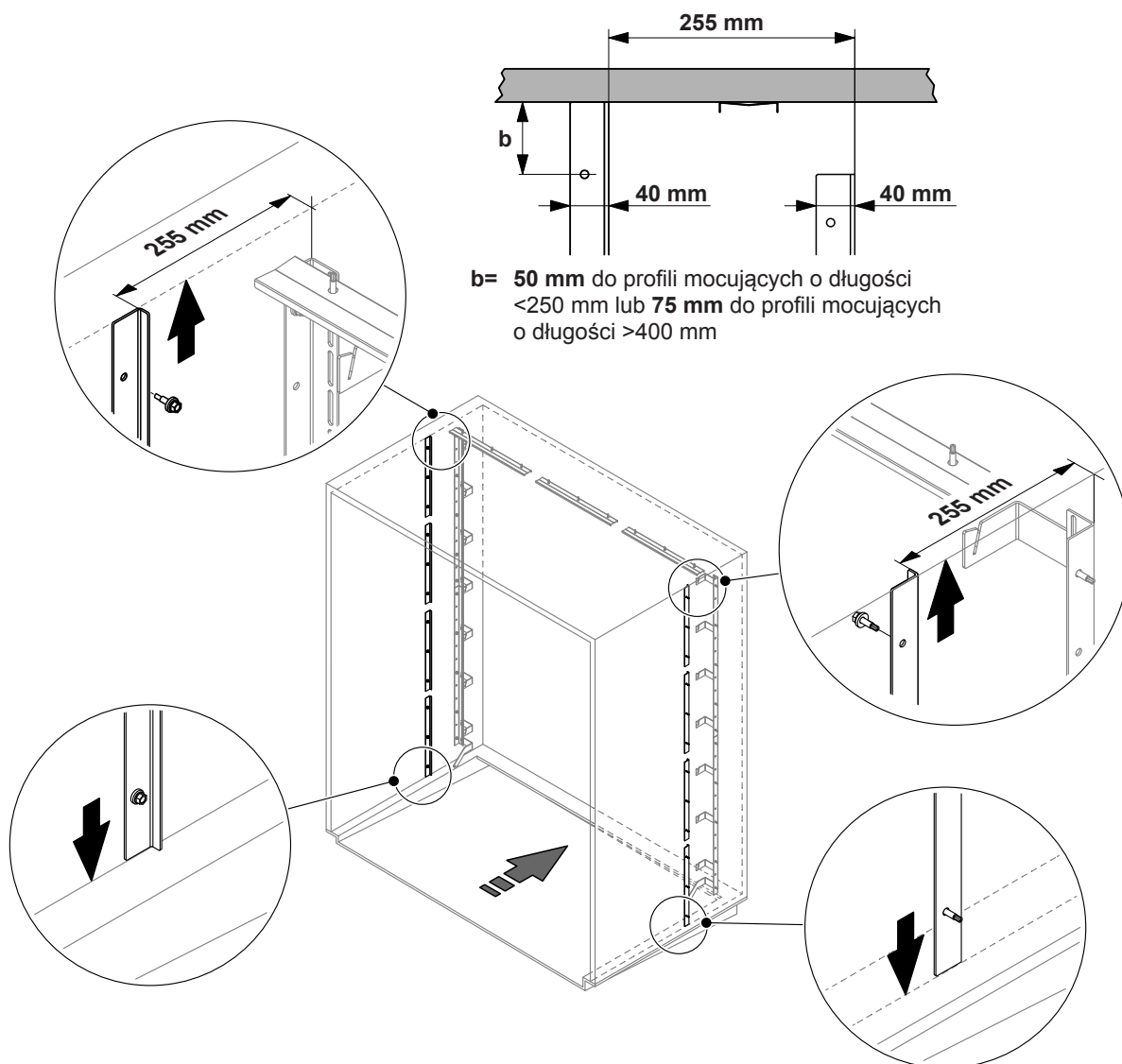
Rys. 9: Montowanie profili mocujących dla bocznych płyt uszczelniających
