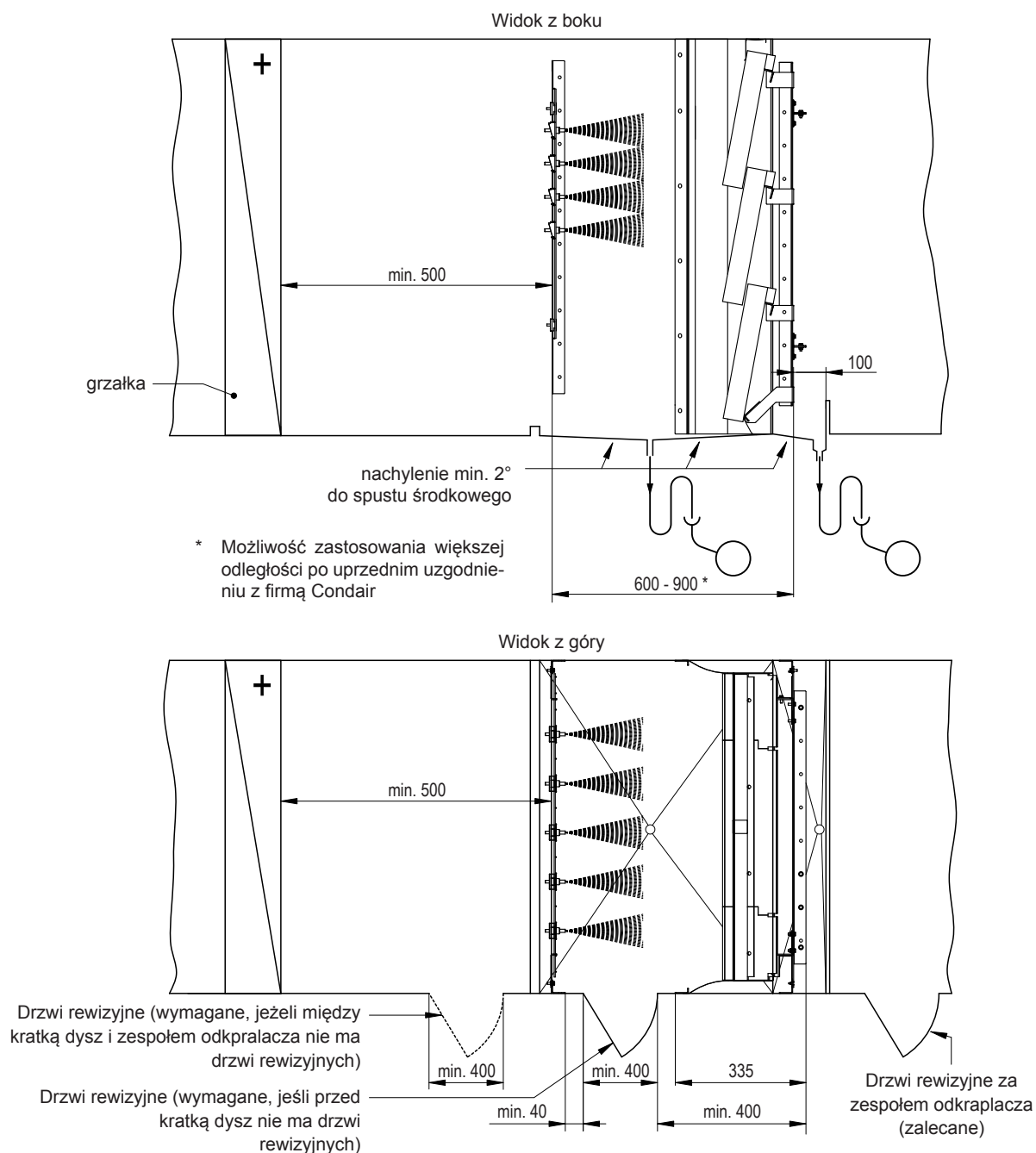
Rys. 2: Umiejscowienie nawilżacza z drzwiami rewizyjnymi między nawilżaczem oraz przed nim i za nim: wymiary w mm
