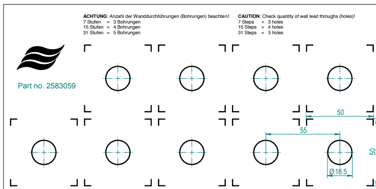
Rys. 31: Szablon do wiercenia otworów przełotowych
