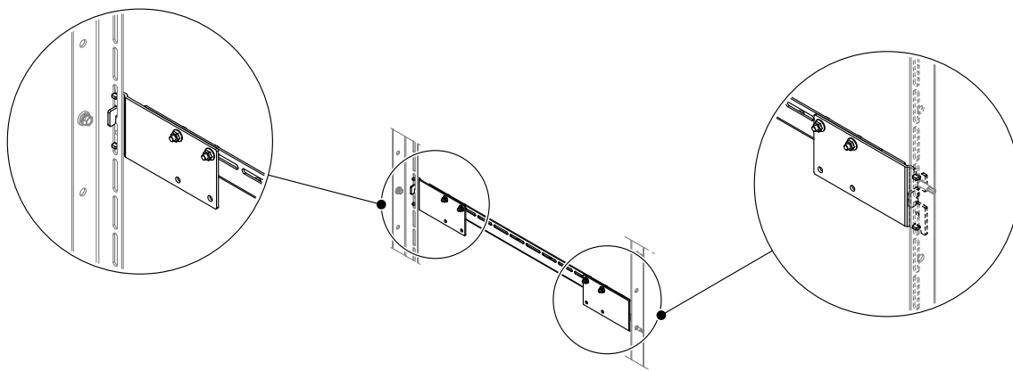
Rys. 15: Montaż wsporników poprzecznych odkraplacza w instalacjach o szerokości do 2100 mm
