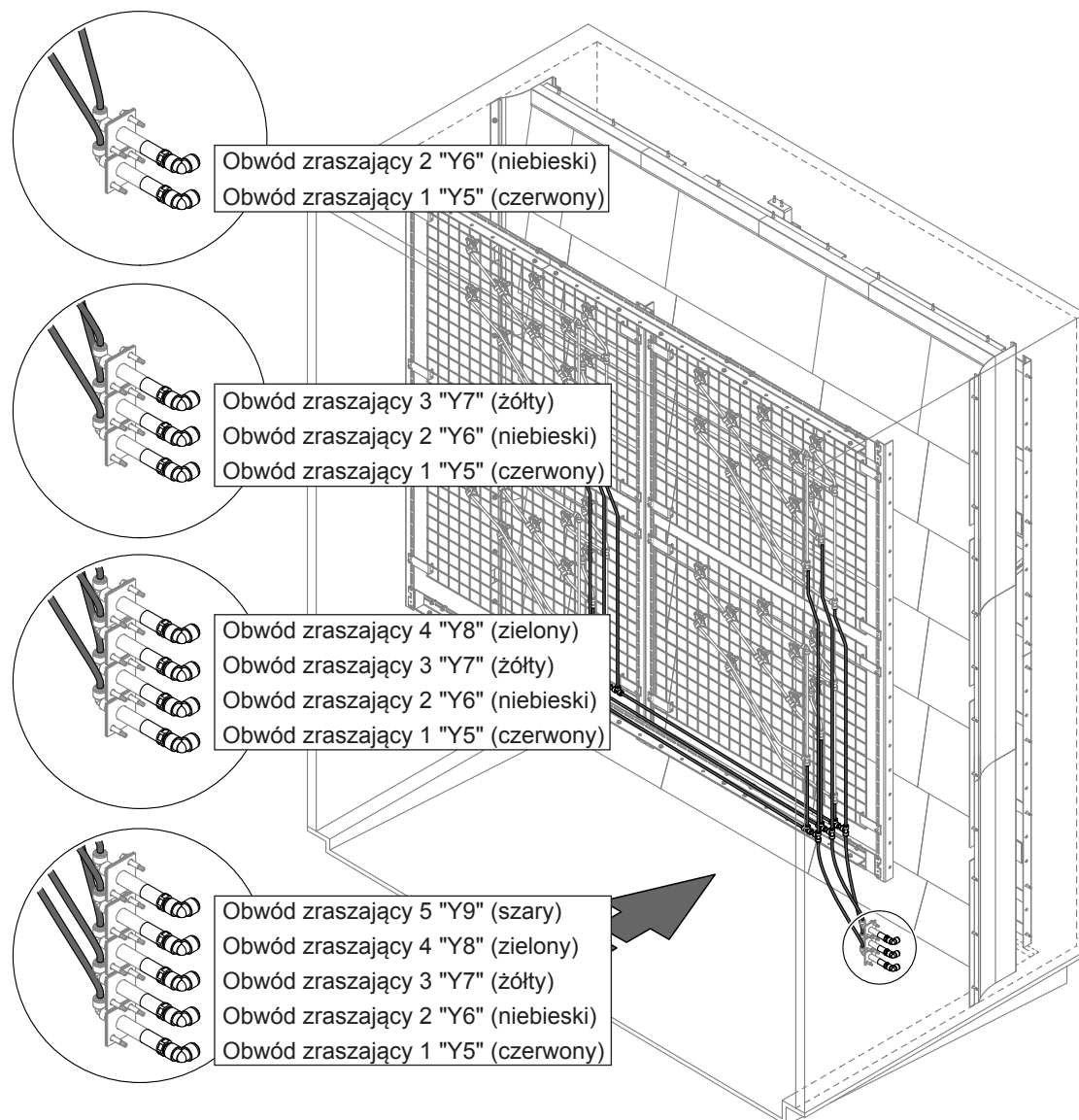
Rys. 33: Podłączanie obwodów zraszające do przepustów
