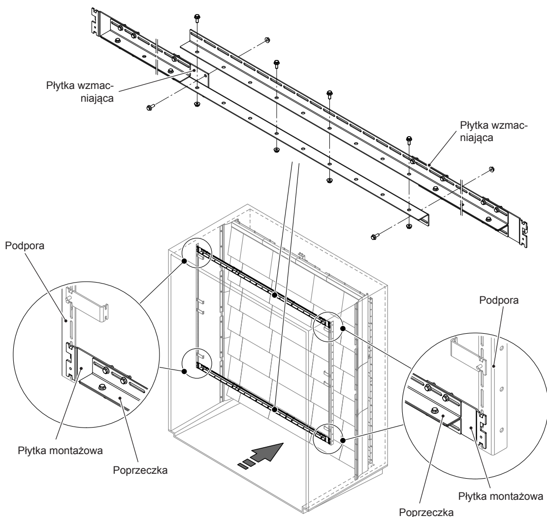
Rys. 26: Montaż poprzeczek
