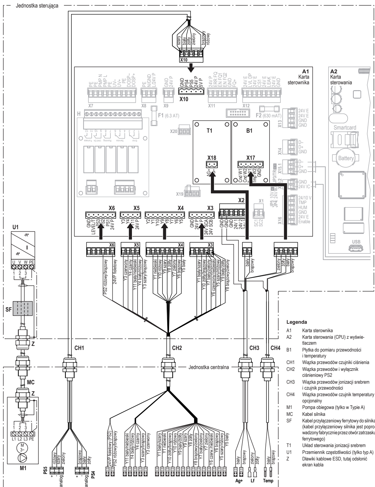
Rys. 39: Schemat połączeń jednostka centralna – jednostka sterująca
