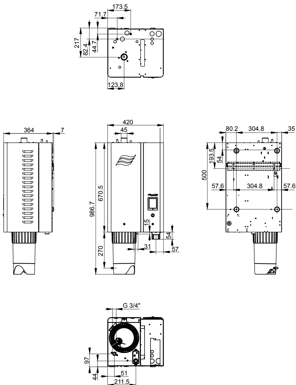
Fig. 29: Rysunek wymiarowy, jednostka mała ("S") (wymiar w mm)
