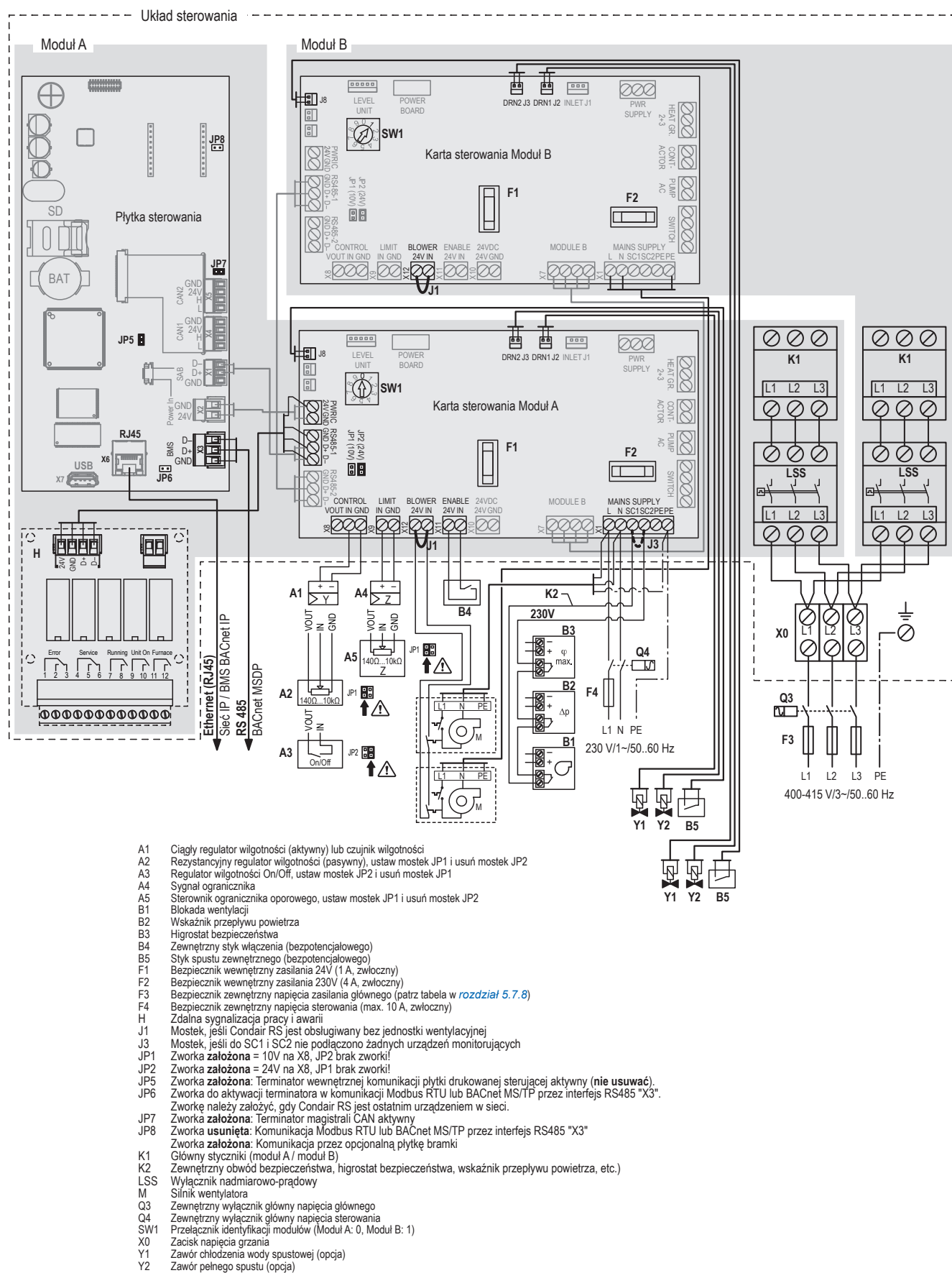
Rys. 29: Schemat połączeń Condair RS 50...80 - jednostki pojedyncze "L" (obudowa podwójna)
